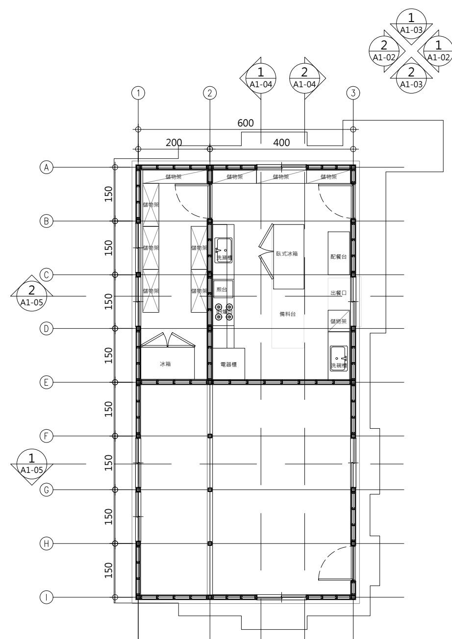
1 一樓平面圖 SCALE: A3=1/100
