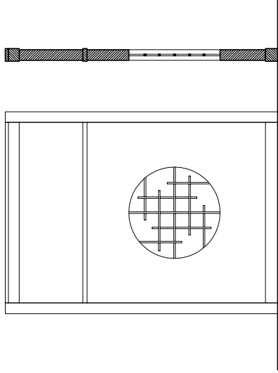
(W2) 立面圖
