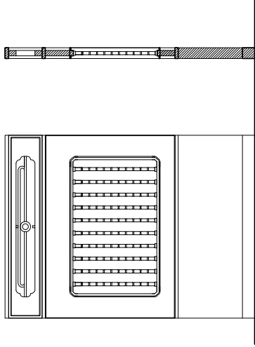
W4 立面圖
