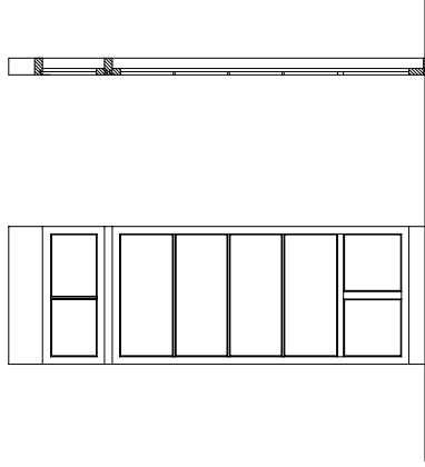
D25 立面圖
