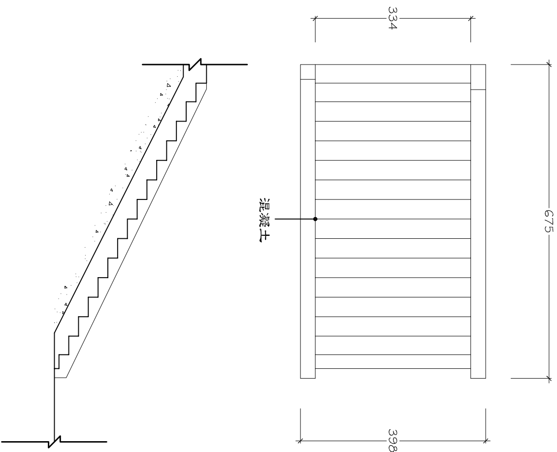
參道3平、剖面圖
