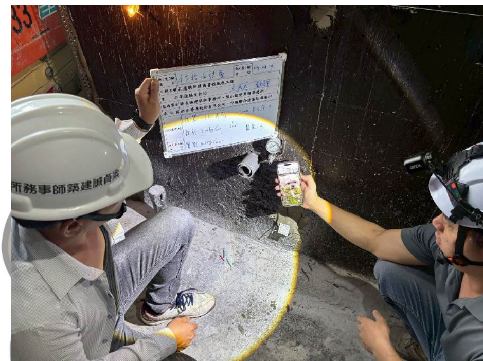
115.04.14 4F給水試壓查驗
