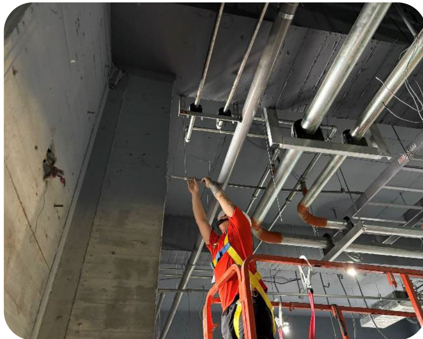
115/4/20-3F 吊管施作
