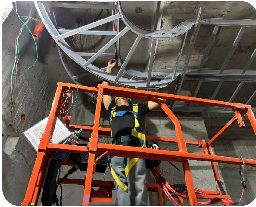
115/4/2-2F 線槽管架組裝
