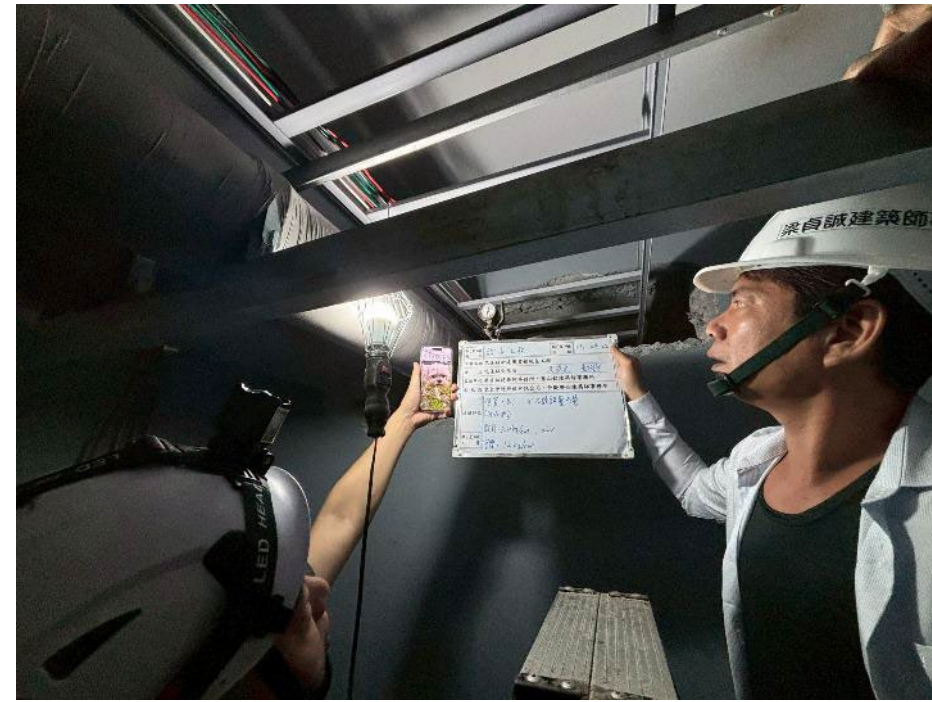
115.04.22 B1污水池給水試壓查驗
